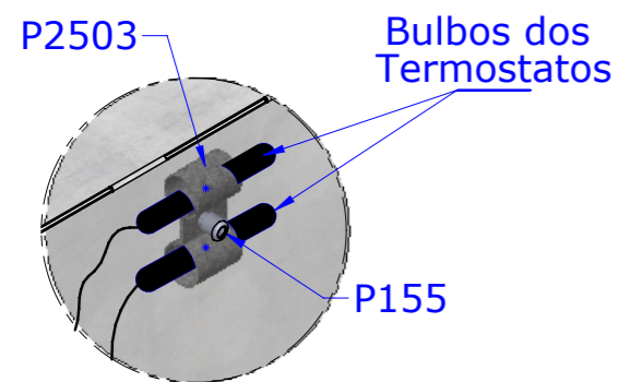
DETALHE P ESCALA 1:2
