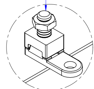
DETALHE Z ESCALA 1 : 1
