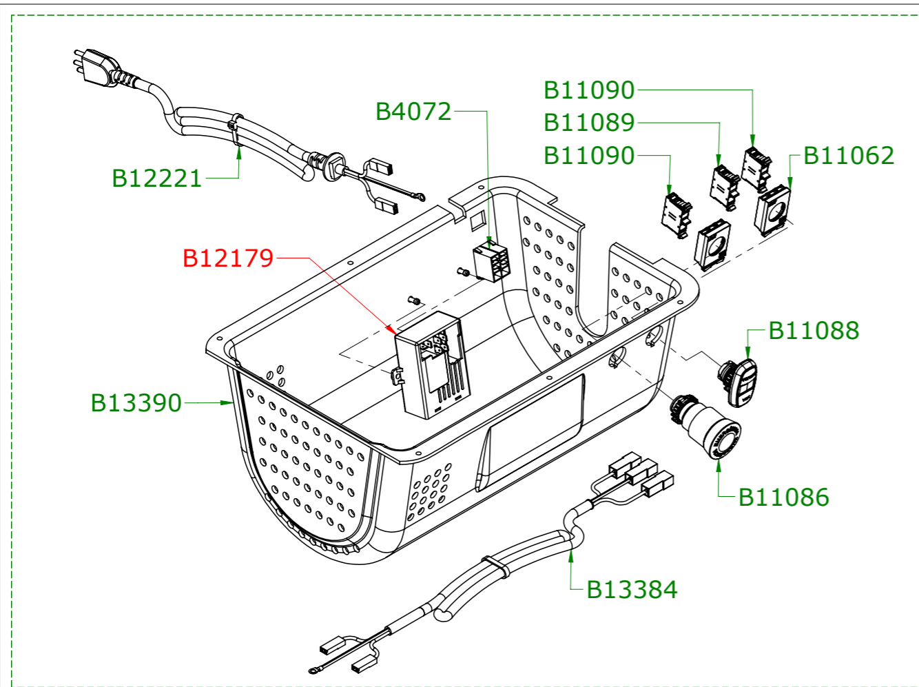
Peças da carenagem montada
