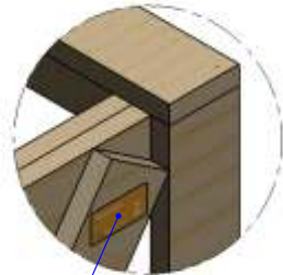
67 DETALHE P ESCALA 1 : 5
