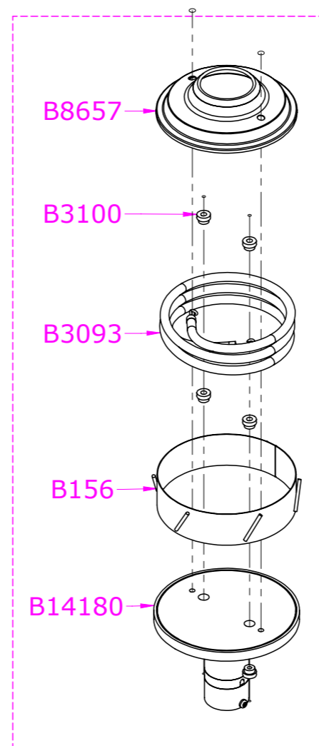
Componentes do conjunto B14181
